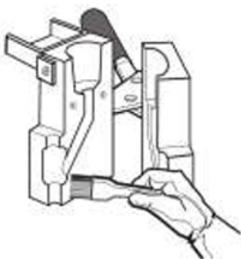
Figura 9: Eliminar los restos de la cámara de soldadura por medio de la brocha
