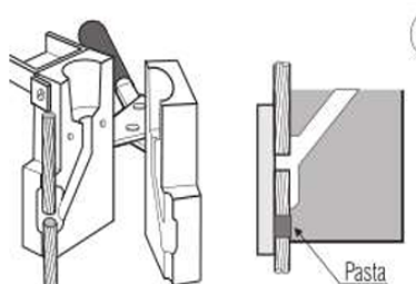
Figura 3: Introducir en el molde los cables a soldar según se muestra en la figura.
