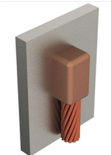
Figura 1: Molde Grafito M-VBC
