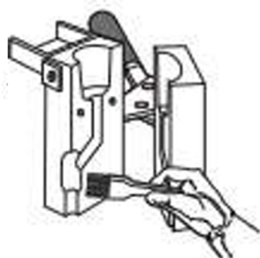
Figura 9: Eliminar los restos de la cámara de soldadura por medio de la brocha
