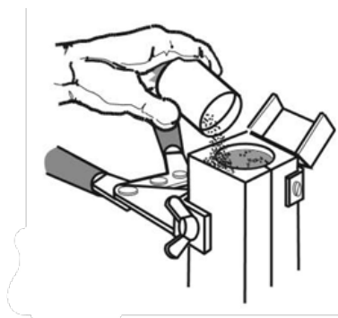
Figura 7: Espolvorear el polvo de ignición sobre la soldadura y depositar aprox. un 25 % sobre el borde del molde
