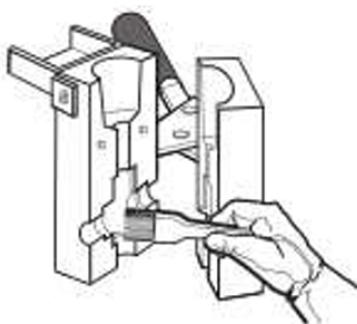
Figura 10: Eliminar los restos de la cámara de soldadura por medio de la brocha
