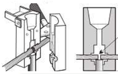
Figura 3: Introducir en el molde los cables a soldar según se muestra en la figura.
