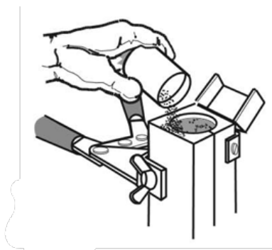
Figura 6: Espolvorear el polvo de ignición sobre la soldadura y depositar aprox. un 25 % sobre el borde del molde
